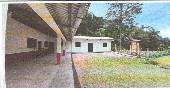
Foto 3: Se observa aplicación de pintura exterir en modulo dos, instalcion eléctrica, fundición de banquetas.
