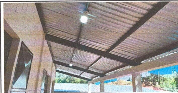
Foto 5: aplicación de pintura en módulo uno, instalaciones electricas, mantenimiento de vigas en modulo dos.
